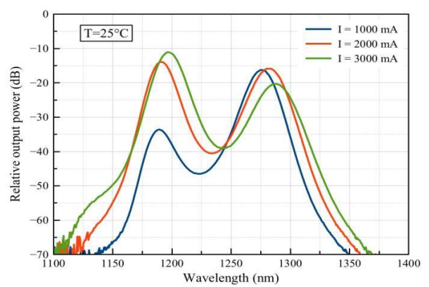
光谱(ASE)
