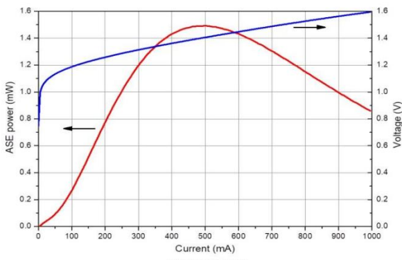
L-I-V 曲线
